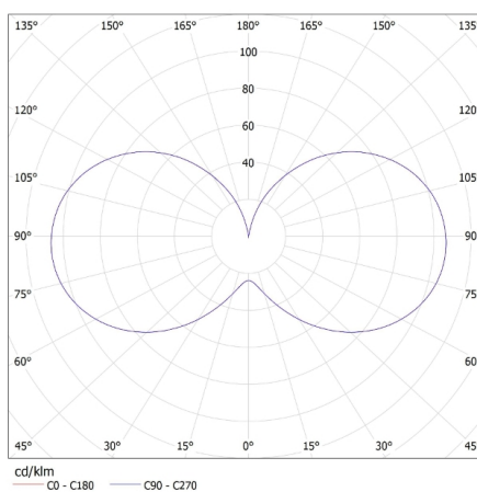
KANLUX S.A. (kat 29622) XLED C35E14 6W-WW-M / LDC (Polar)
