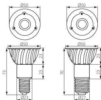
POWER-LED3W E14
